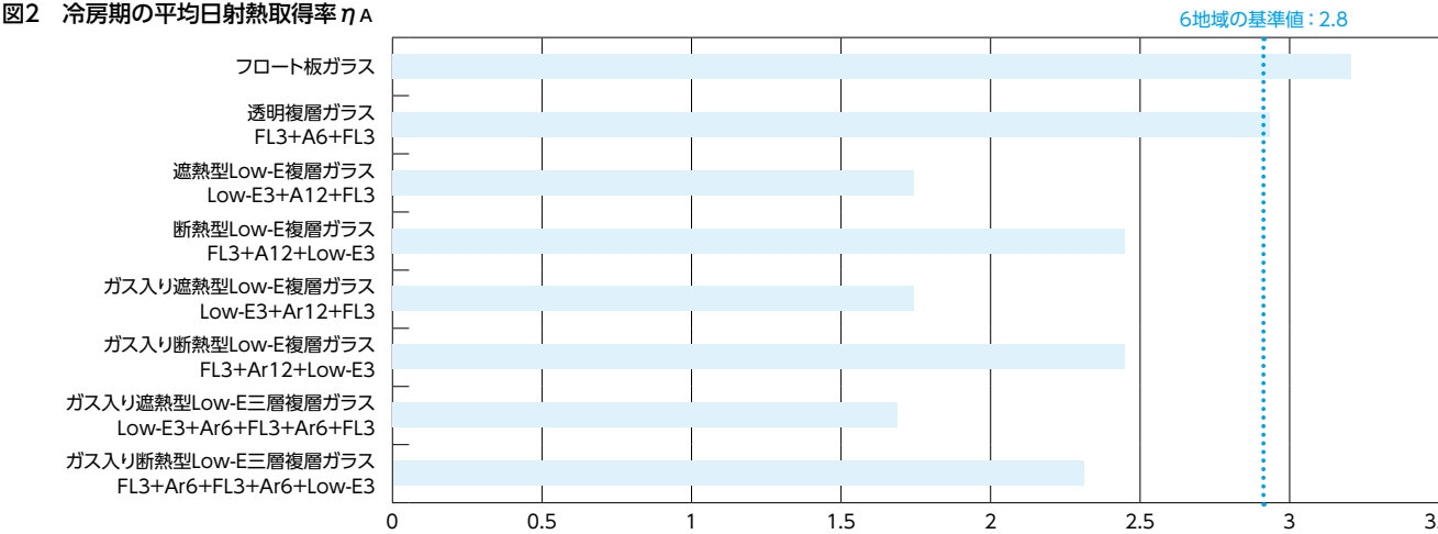
図2 冷房期の平均日射熱取得率 \eta_A
