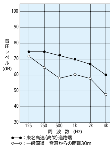
図15 道路騒音
