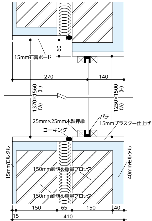
図7 開口部調整壁の垂直断面
