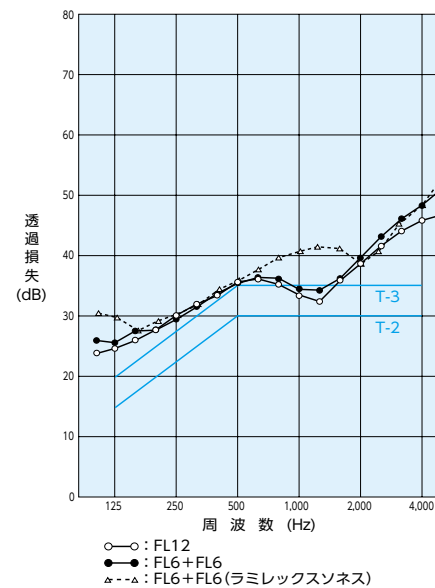
図12 各種ガラスの遮音性能の比較
