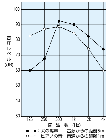
図19 環境騒音
