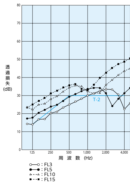
図11 二重ガラスの遮音性能の比較
