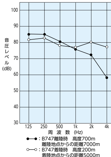
図17 航空機騒音
