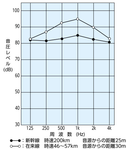
図16 鉄道騒音
