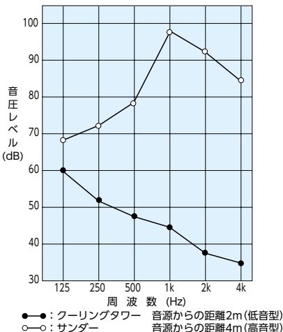
図18 特殊騒音
