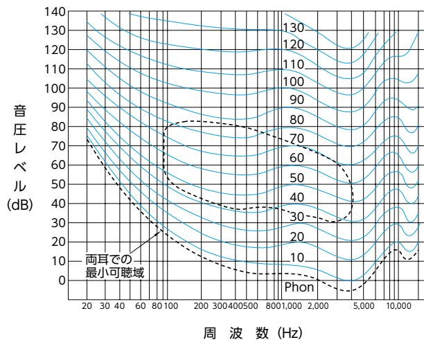
図1 等ラウドネス曲線
