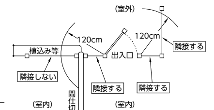
図2 間仕切壁がある場合の出入口に隣接するガラス、隣接しないガラスの例
