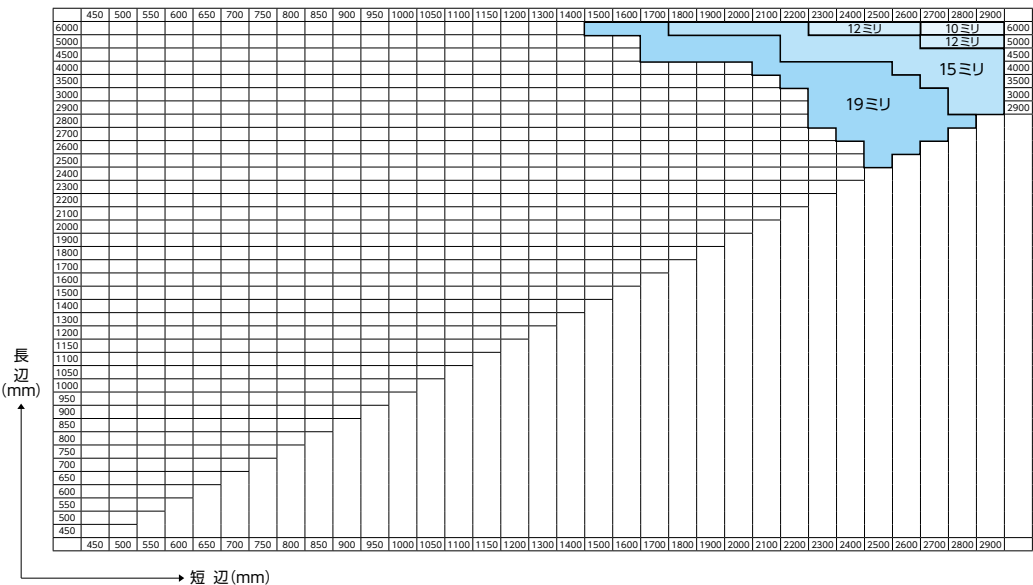
別表6 落下高さ75cmで割れないガラス (フロート板ガラス) 注) 長辺6000mm以上の場合は6000の欄を適用する
