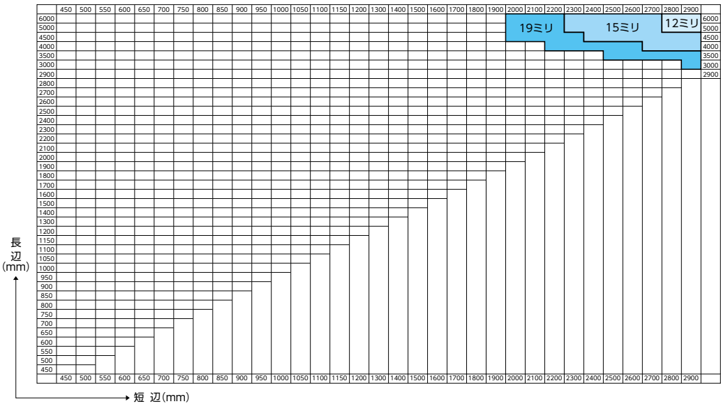
別表12 落下高さ120cmで割れないガラス (フロート板ガラス) 注) 長辺6000mm以上の場合は6000の欄を適用する
