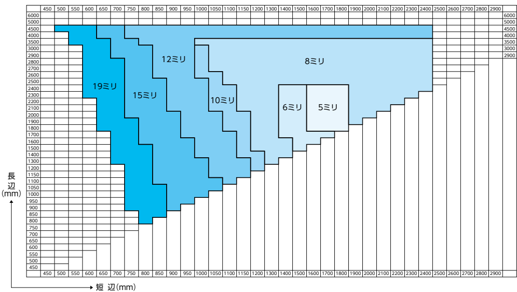
別表8 落下高さ75cmで割れないガラス (強化ガラス)
