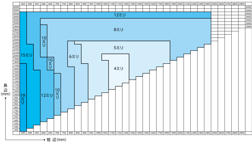
別表3 落下高さ30cmで割れないガラス (強化ガラス)
