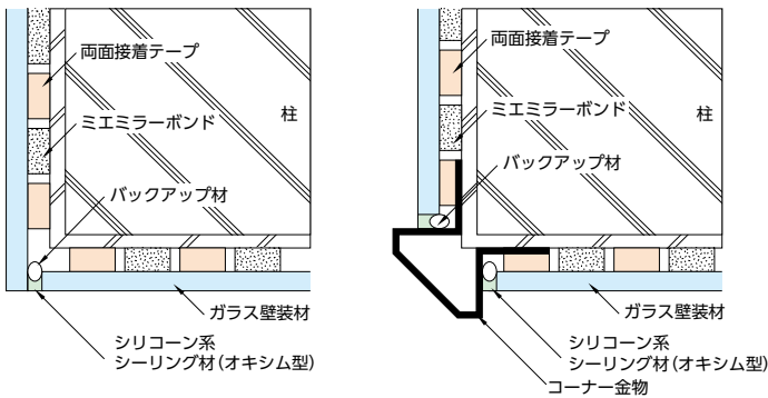
出隅施工例
