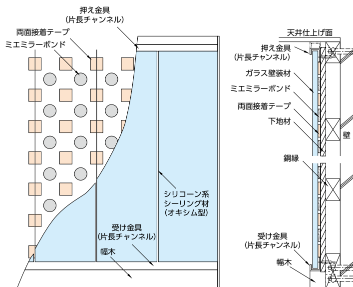
④ 大板接着受け金具方法
