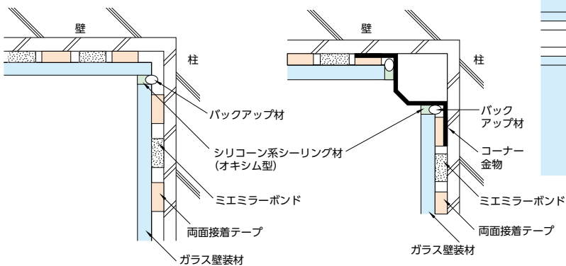
入隅施工例
