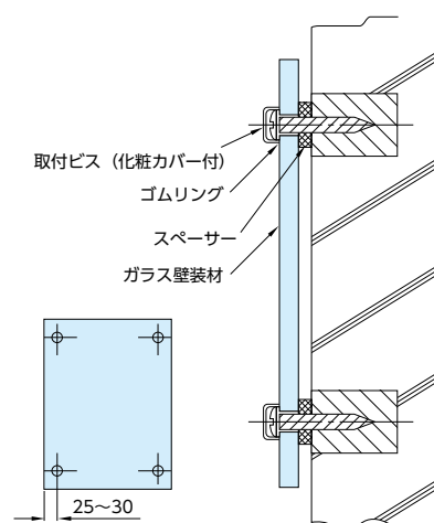
② ビス止め方法
