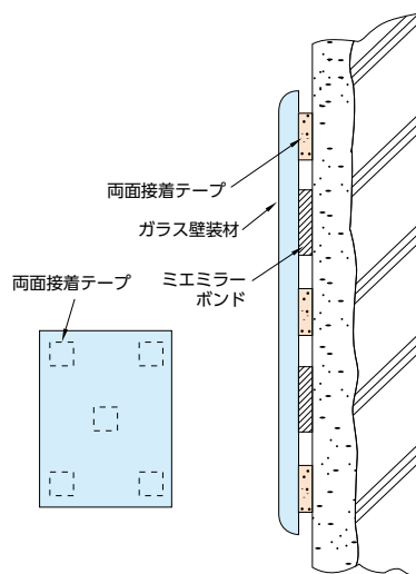
① 接着方法
