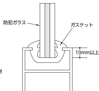
図2 ガスケットの例
