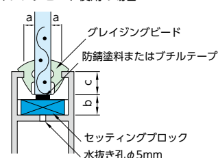
グレイジングビード使用の場合
