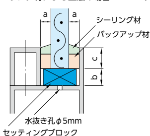
シーリング材による工法の場合
