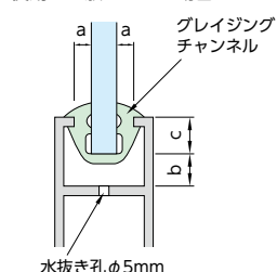
グレイジングチャンネル使用の一般サッシの場合
